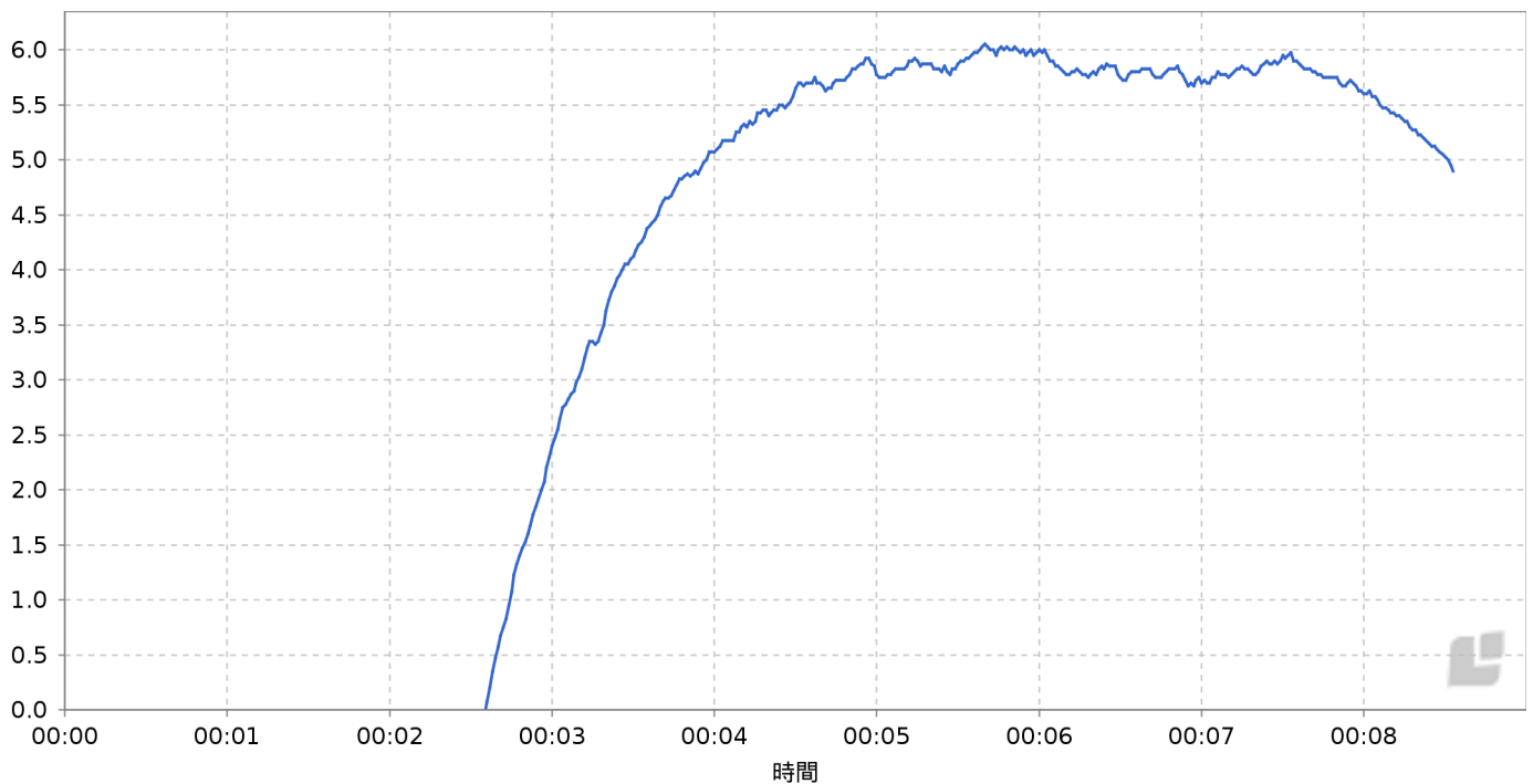
— 豆の温度
